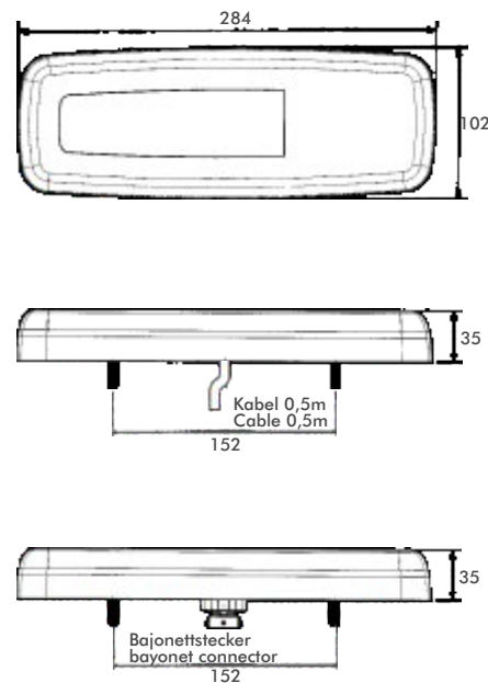
40 057 502 seitl. Kennzeichn./ lat. Numberplate Lamp
